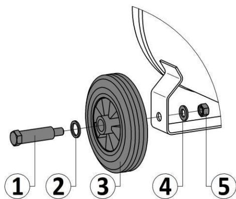
1 - Болт 2 - Шайба 3 - Колесо 4 - Гайка M12 5 - Шайба 12 Рисунок 1
