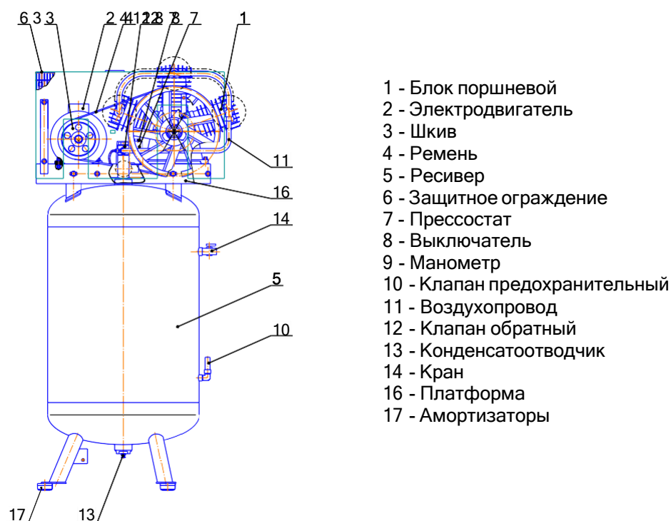
Рисунок 10 - Общий вид компрессора СБ4/Ф-270.LB40B
