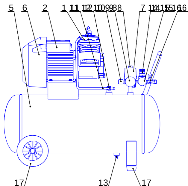
Рисунок 9 - Общий вид компрессора СБ4/С-50.J2047В
