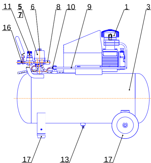
Рисунок 6 - Общий вид компрессора СБ4/С-50.J1047В
