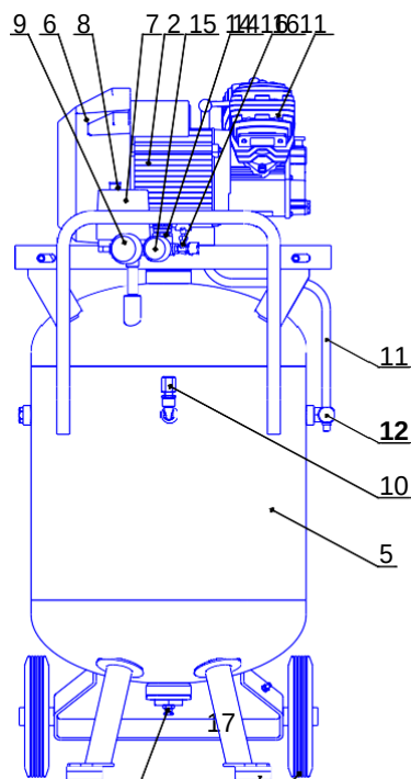
Рисунок 11 - Общий вид компрессора СБ4/С-100.Ј2047ВВ
