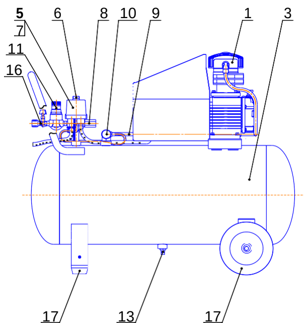
Рисунок 8 - Общий вид компрессора СБ4/С-50.J1048В
