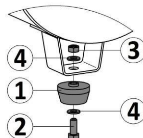
1 - Амортизатор 2 - Болт M10x25 3 - Гайка M10 4 - Шайба 10 Рисунок 3
