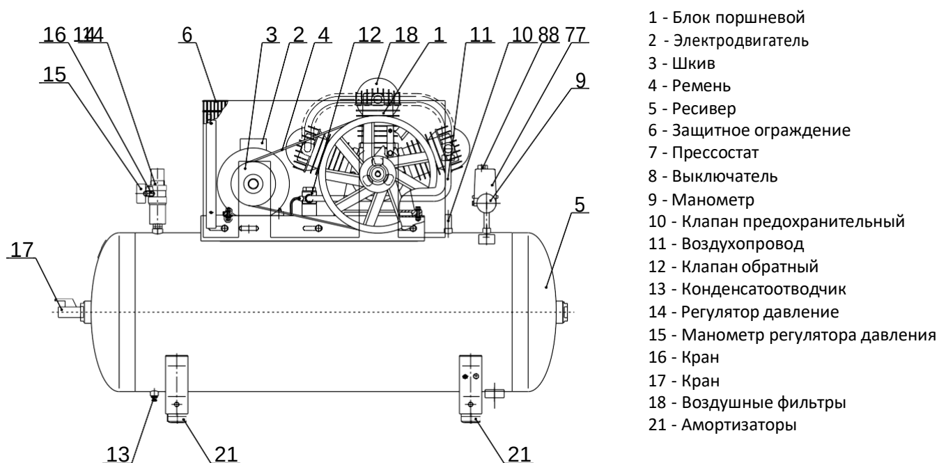
Рисунок 4 - Общий вид компрессора СБ4/Ф-100.LB75
