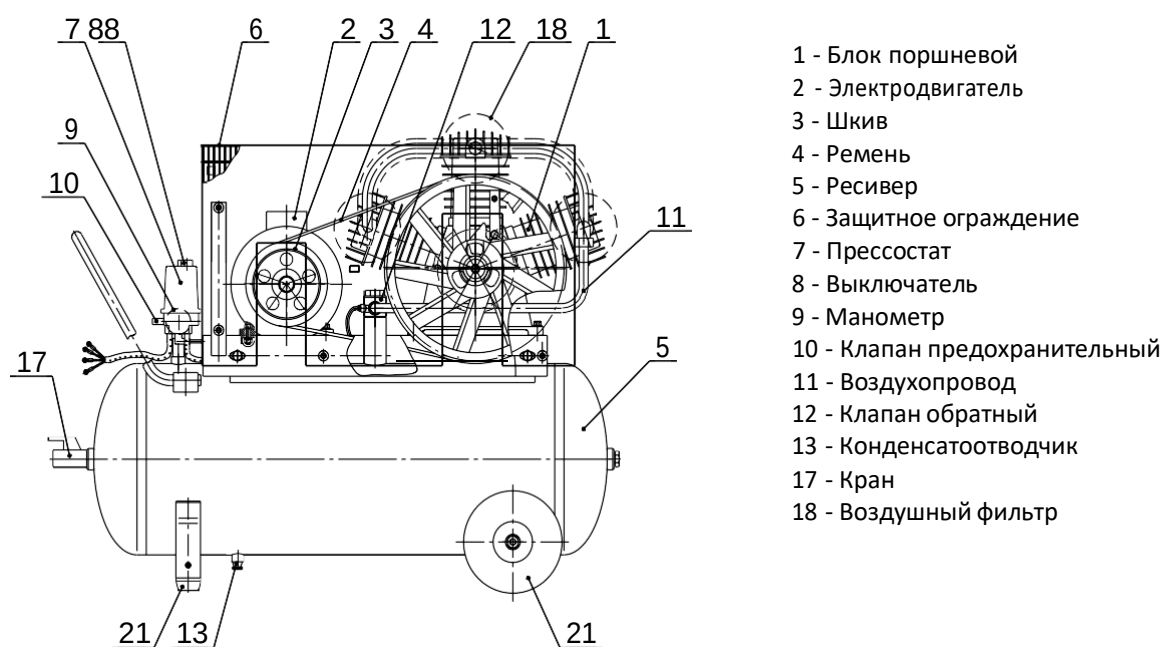
Рисунок 4 - Общий вид компрессора СБ4/Ф-100.LB75
