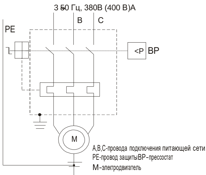
Рисунок А.1 - Схема электрическая принципиальная компрессоров CB4/C-100.LB75, CB4/Ф-270.LB75, CB4/Ф-270.LB75B, CB4/Ф-500.LB75
