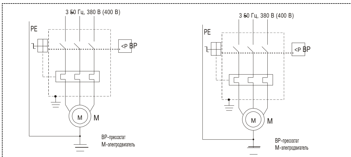
Рисунок А.2 – Схема электрическая принципиальная компрессора CB4/Ф-500.LB75TB
