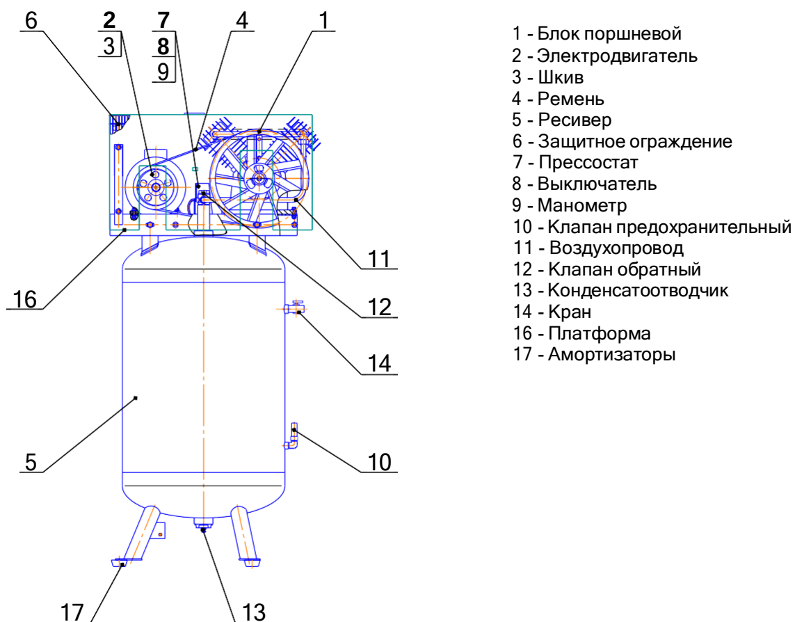
Рисунок 6 - Общий вид компрессора СБ4/Ф-270.LB50B
