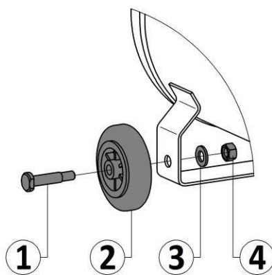
1 - Болт 2 - Колесо 3 - Шайба 10 4 - Гайка M10 Рисунок 2
