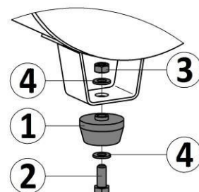
1 - Амортизатор 2 - Болт M10x25 3 - Гайка M10 4 - Шайба 10 Рисунок 3
