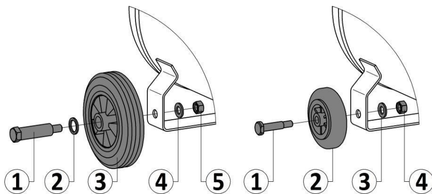
1 - Болт 2 - Шайба 3 - Колесо 4 - Гайка M12 5 - Шайба 12 Рисунок 1
